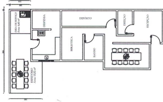
PLANTA BAIXA DE REFORMA ESCALA 1/50
